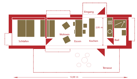
Offenes Modul Pergola + Würfelhaus
